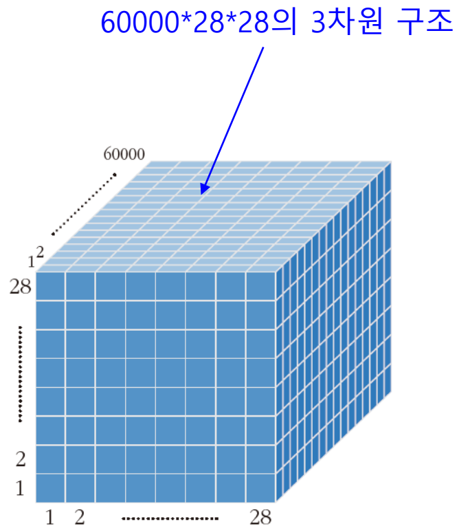
(a) MNIST의 x_train 텐서
