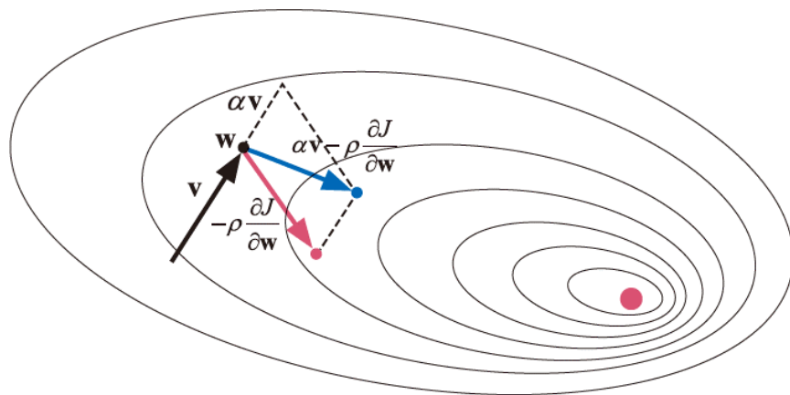
그림 5-15 모멘텀의 원리와 효과
