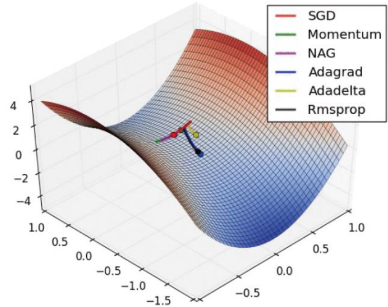
그림 5-17 옵티마이저에 따른 수렴 특성(출처: https://cs231n.github.io/neural-networks-3 )
