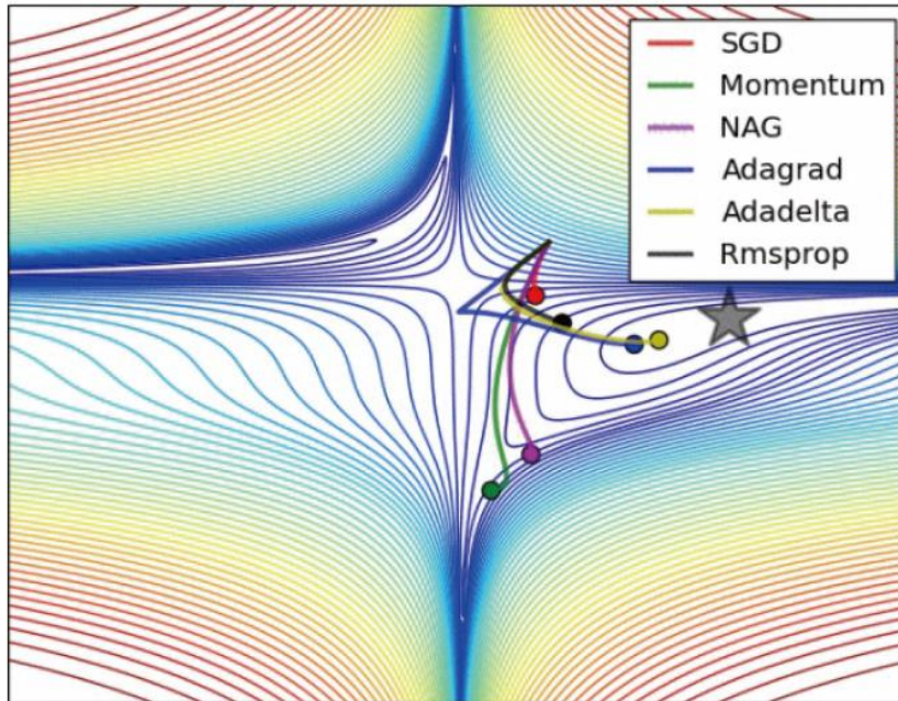
그림 5-17 옵티마이저에 따른 수렴 특성(출처: https://cs231n.github.io/neural-networks-3 )
